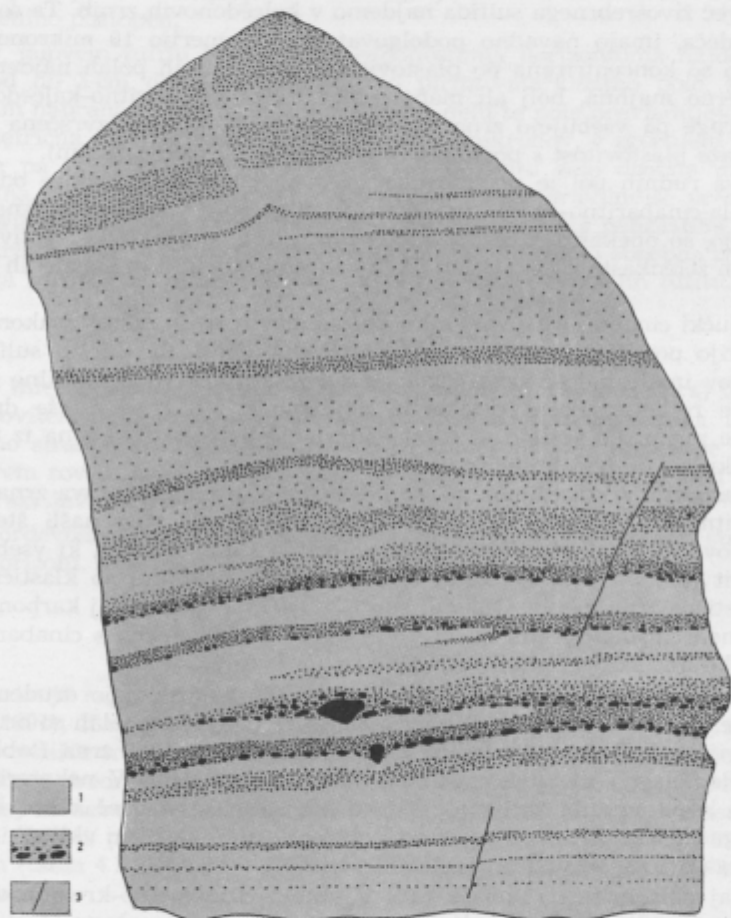
Sl. 2. Živosrebrna ruda iz rudnega telesa Kropač kaže plastovitost s postopno zrnnavostjo. \frac{1}{2} naravne velikosti
